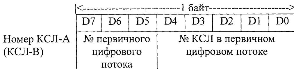
Рисунок 5. Распределение бит в третьем и четвертом байтах
