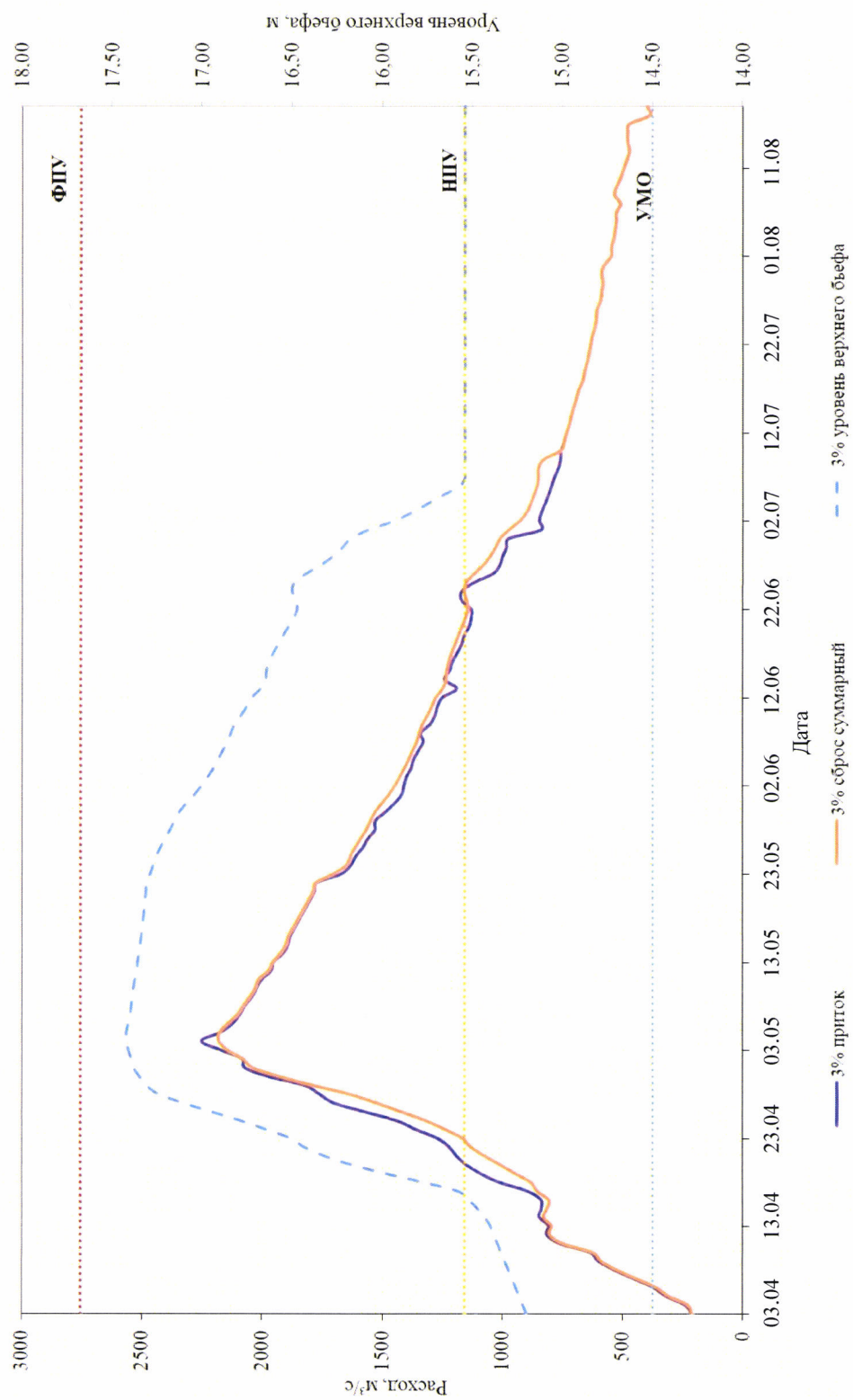
График пропуска половодья обеспеченностью 3%
