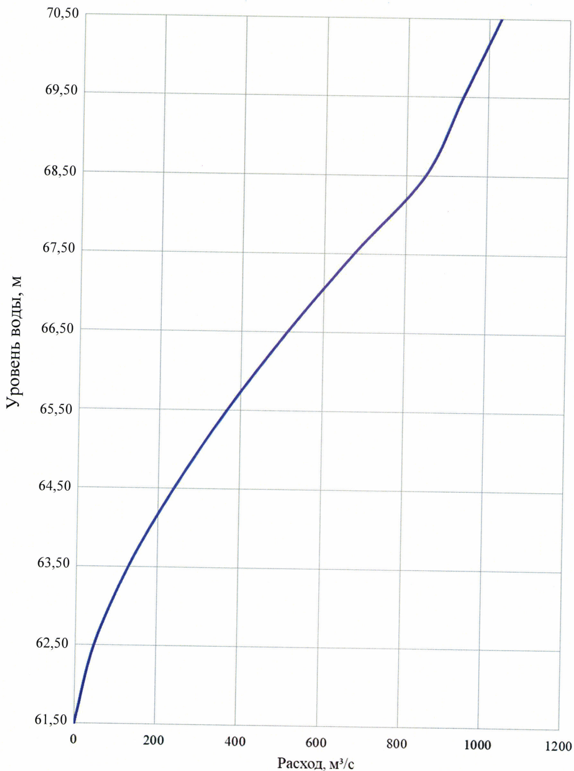
Кривая пропускной способности водосброса Кривопорожского гидроузла
