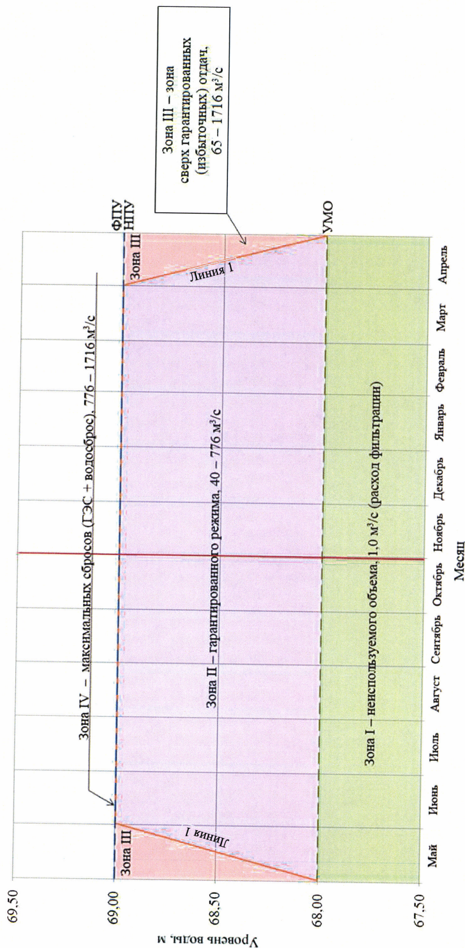
Диспетчерский график работы Кривопорожского водохранилища
